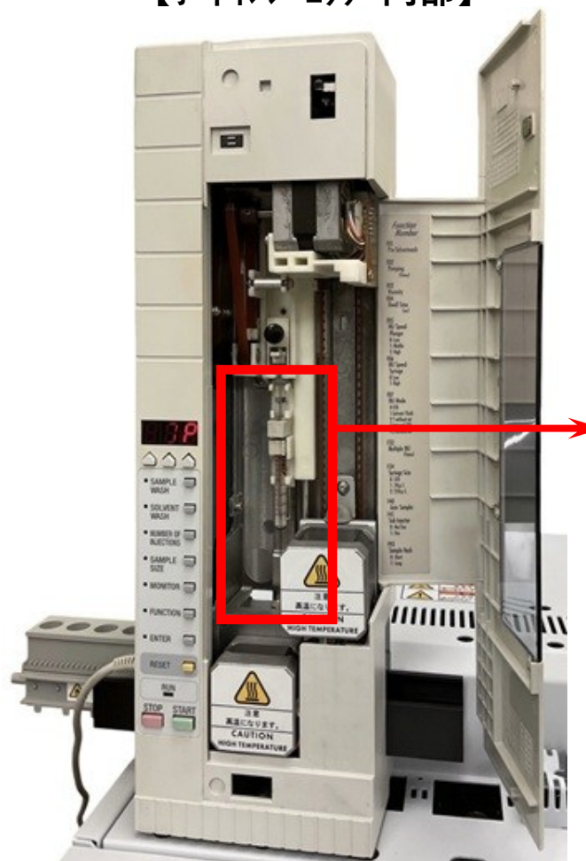
【オートインジェクター-内部】
