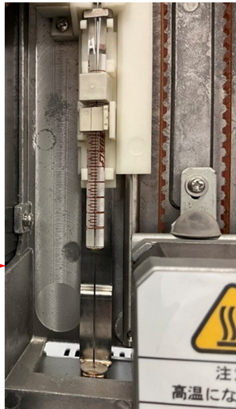
【オートインジェクター-内部拡大=シリンジ部】
