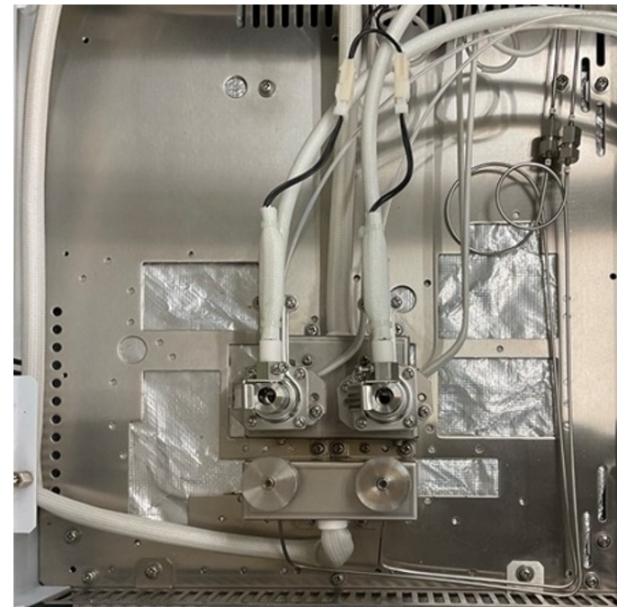
【注入口と検出器(FID)】
