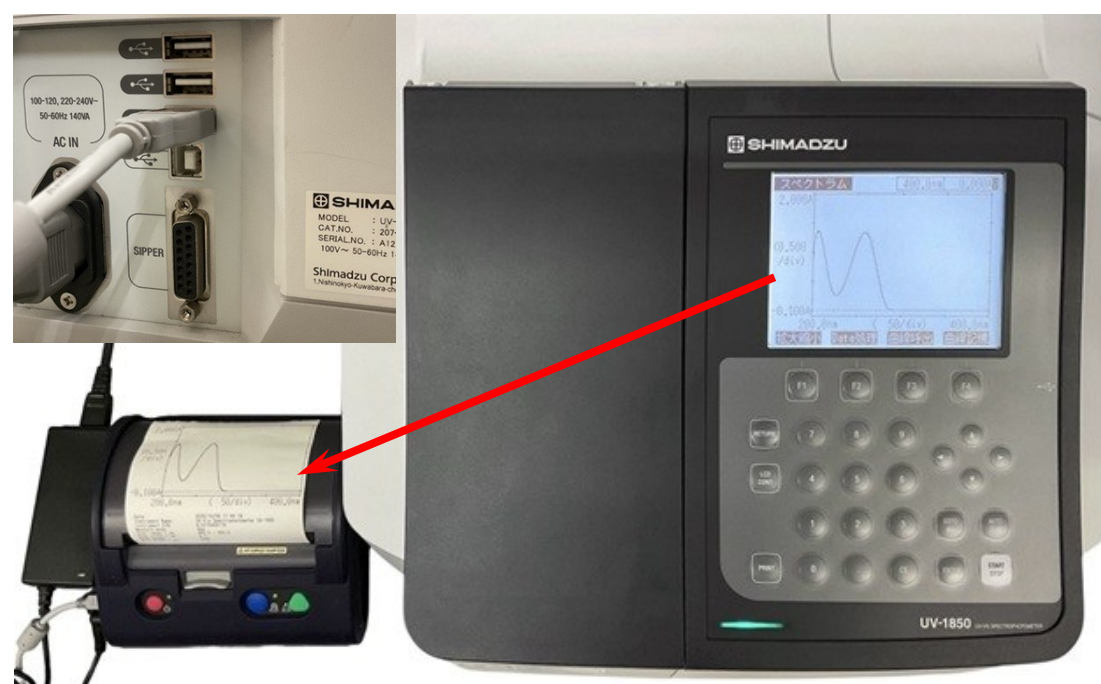
【島津UV-1850～接続使用例】
