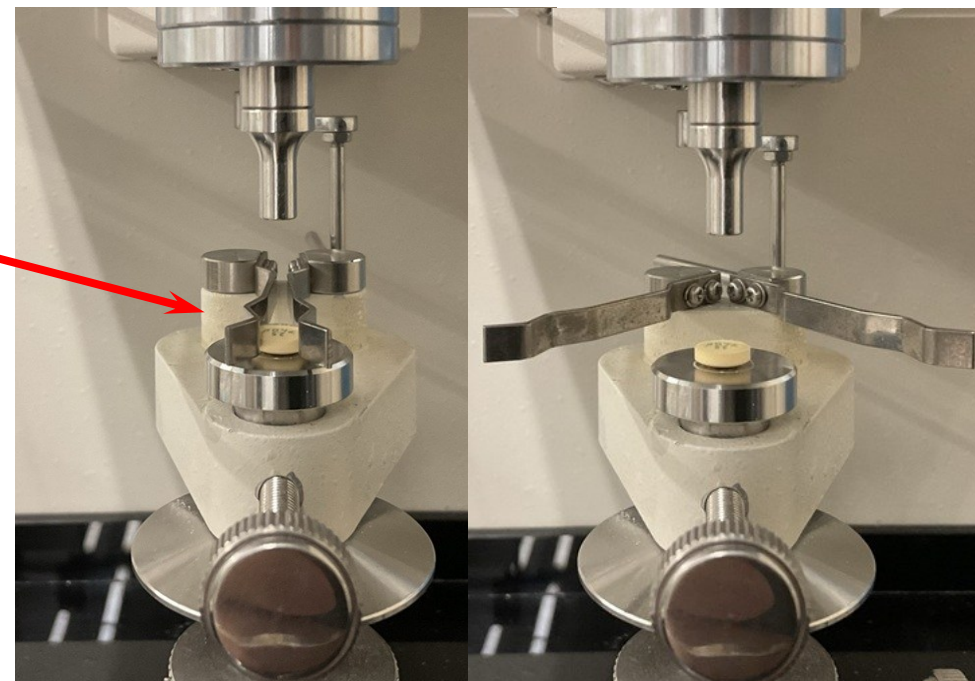
【錠剤硬度測定部拡大】
