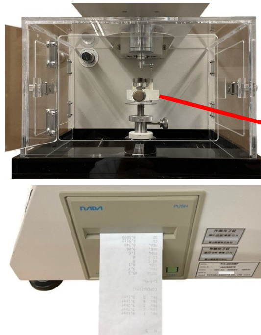
【測定室、プリンター部】
