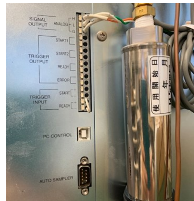
【装置背面端子】
