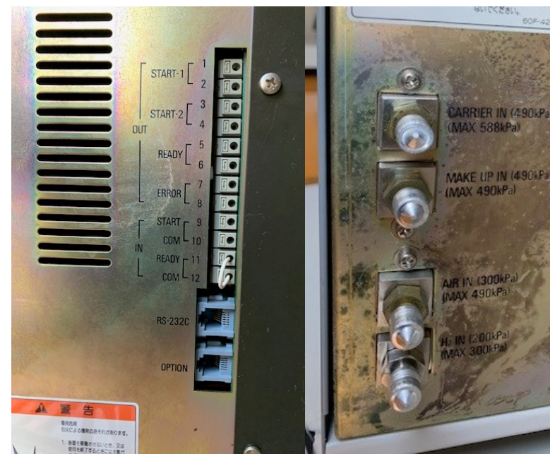
【装置背面端子およびガス接続口】
