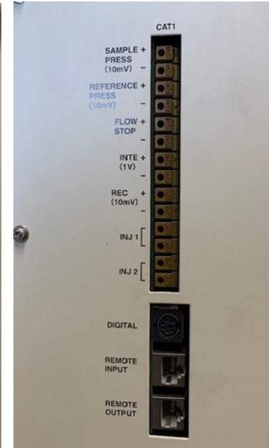
【背面端子】
