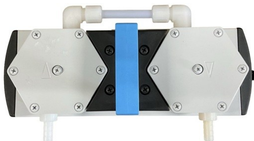
【装置上面】
