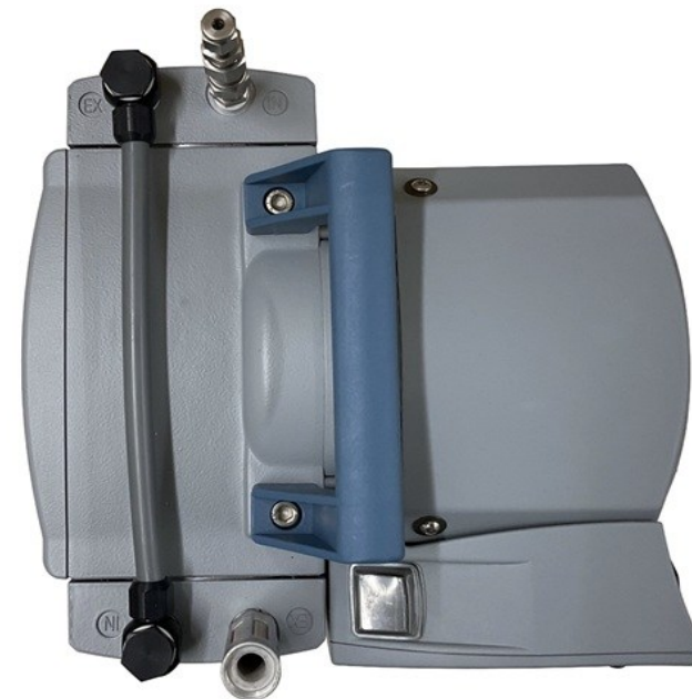
【装置上面】
