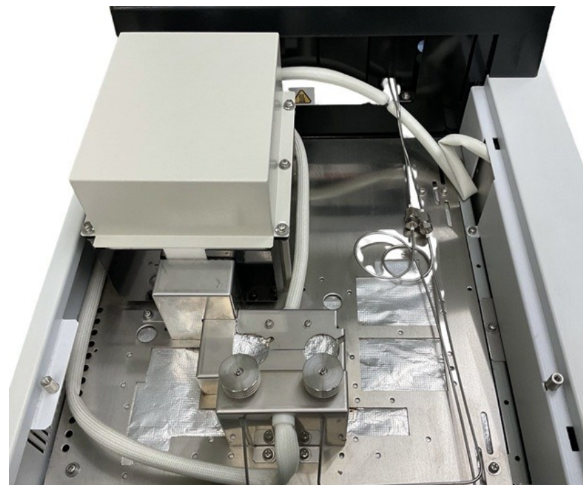
【注入口と検出器(TCD)】
