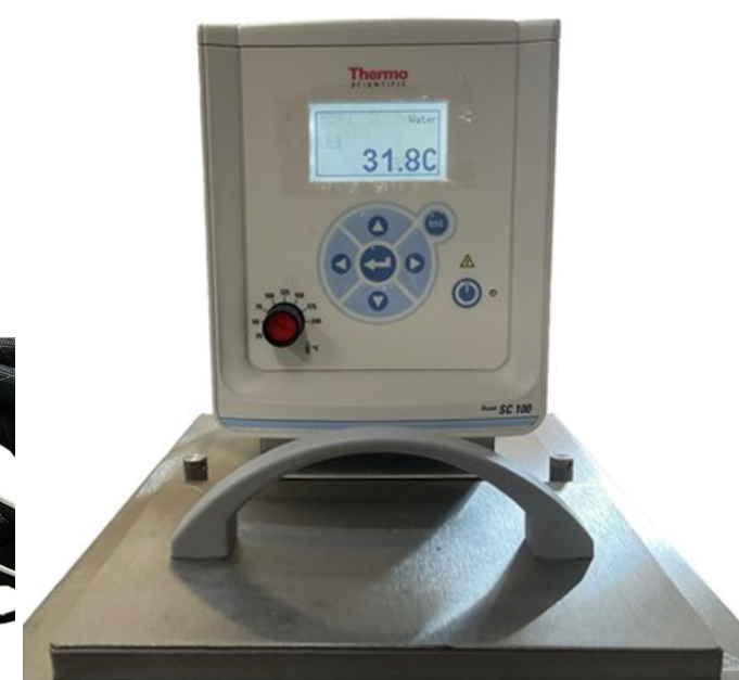
【水槽部-拡大2】
