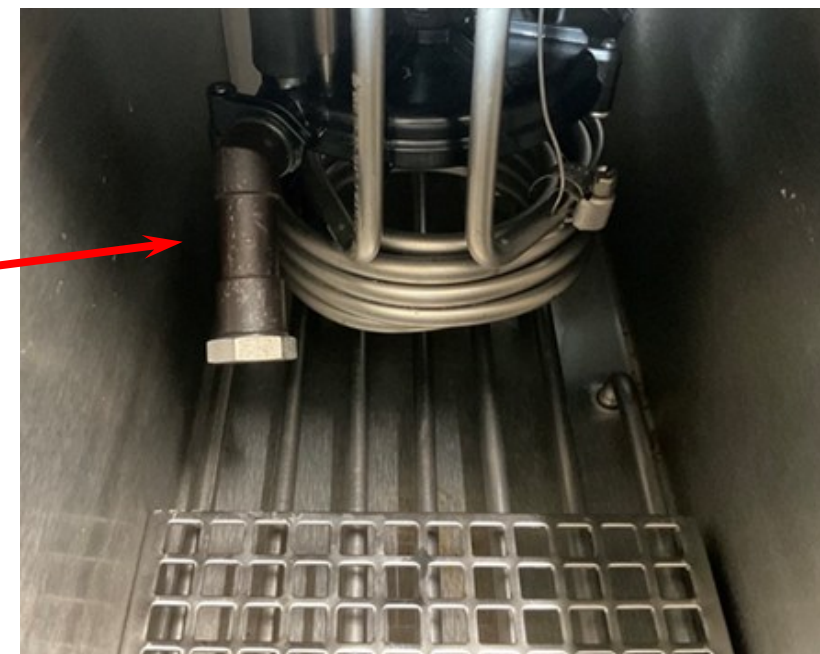
【水槽部-拡大2】
