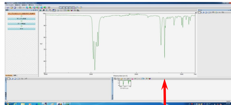
【ATR装置測定面拡大および測定例チャート(PP)】
