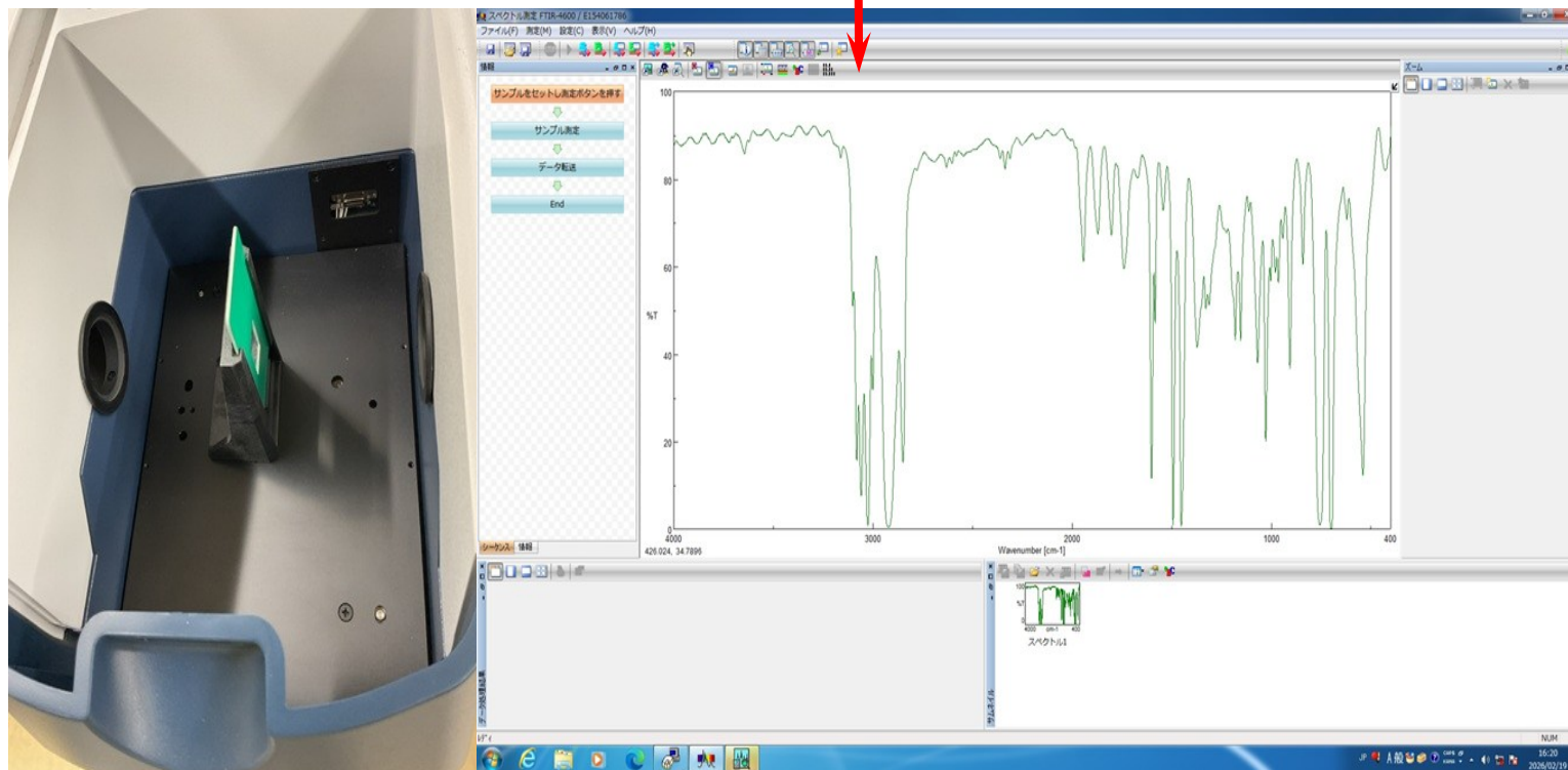
【FT-IR装置透過法PS-FILM測定例】
